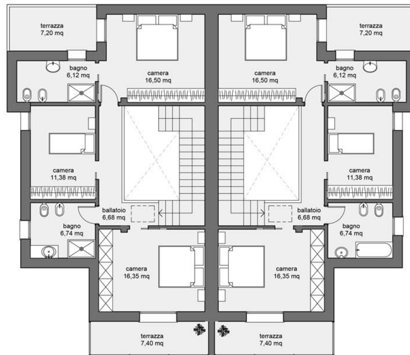
PIANO PRIMO
