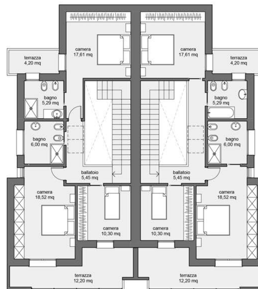
PIANO PRIMO
