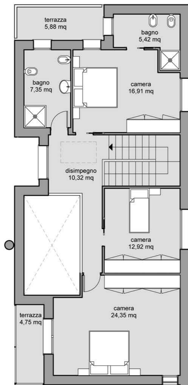
PIANO PRIMO
